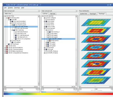
Scalasca
