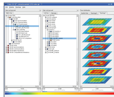
Scalasca
